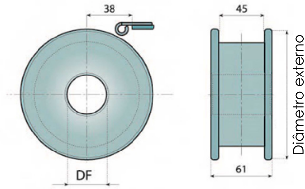
POLIA DE RETORNO USINADA
